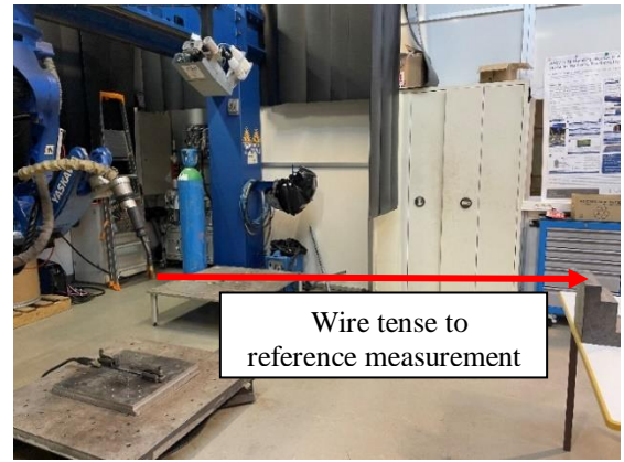
Fig. 3. CMT setup
