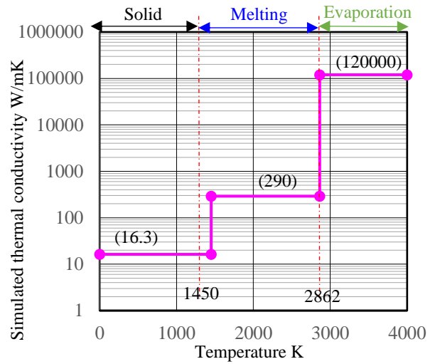
(d) Simulated thermal conductivity B for top region
